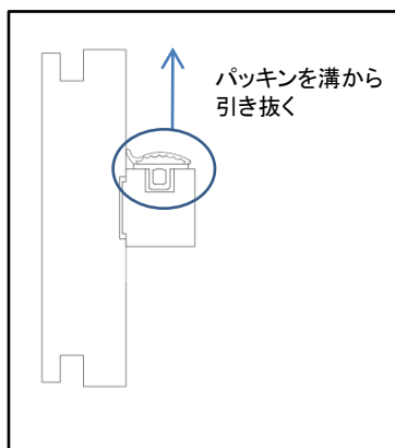
イメージ図(枠断面図)
