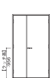
正面図
