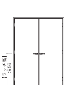
正面図
