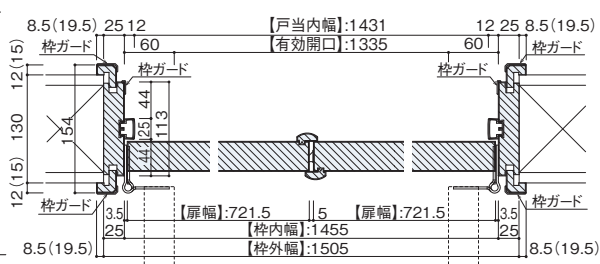
縦枠断面図
