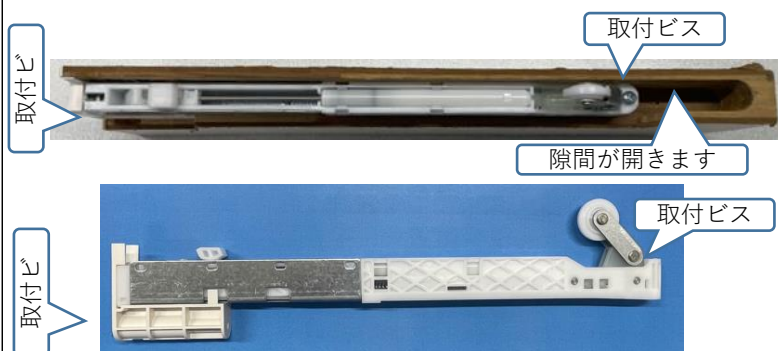
現行ラクラクローズ金具
