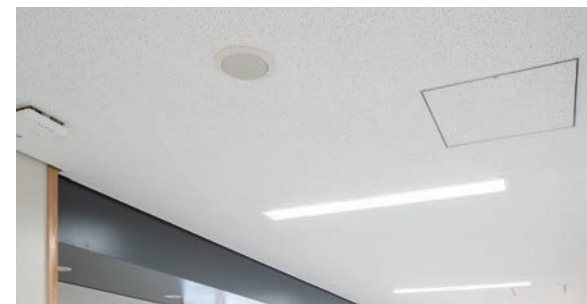
耐震天井工法：ダイケンハイブリッド天井 天井材：ロックウール化粧吸音板 ダイロートン ギンガ4 DAIKEN © DAIKEN CORPORATION 2021.07
