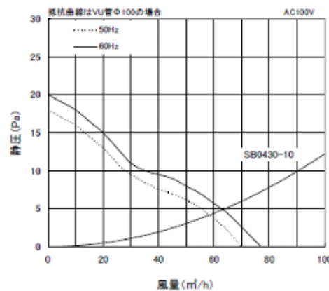
P-Q特性図
