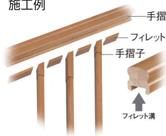
施工例
