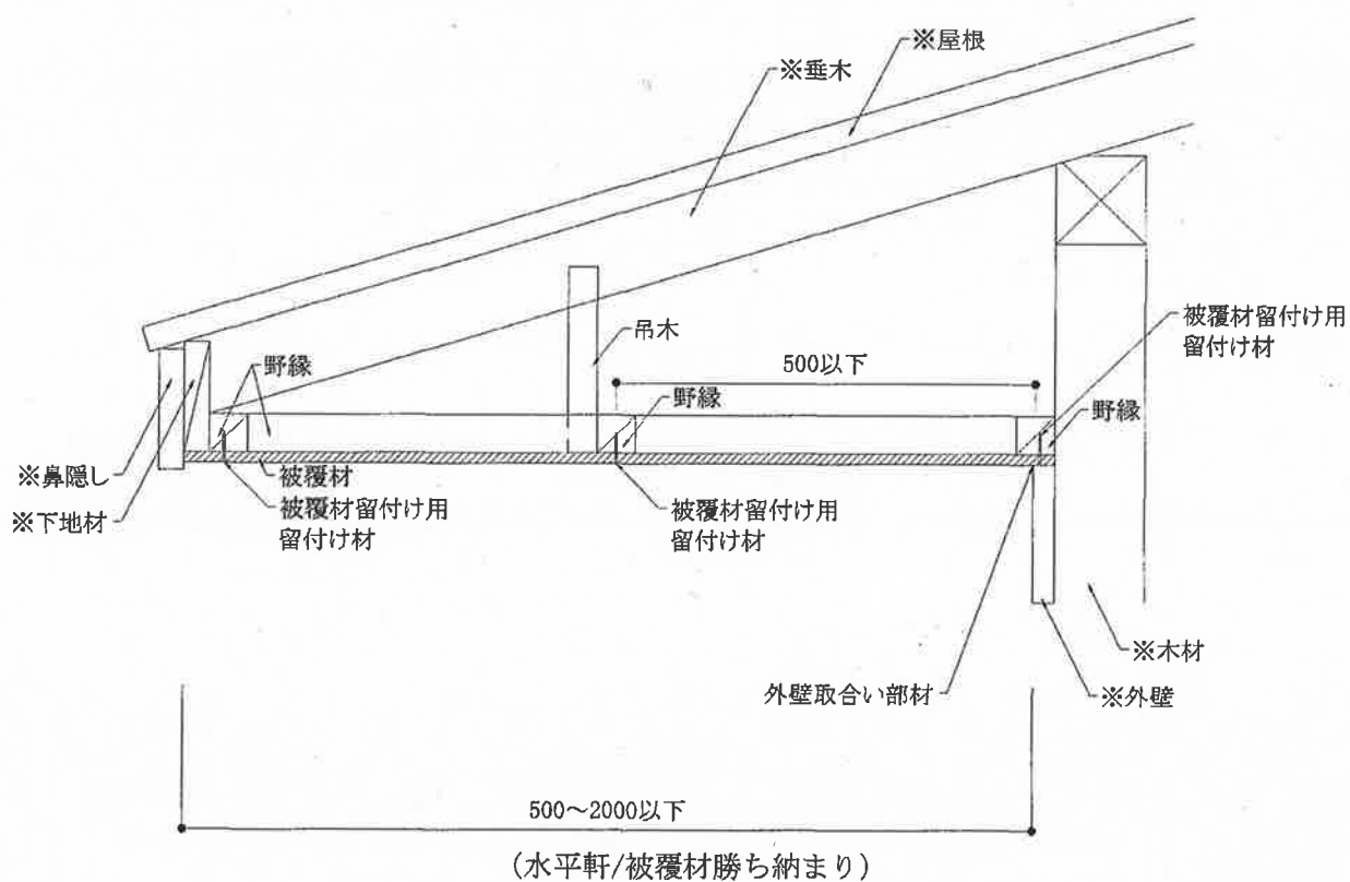
図 3 構造説明図
