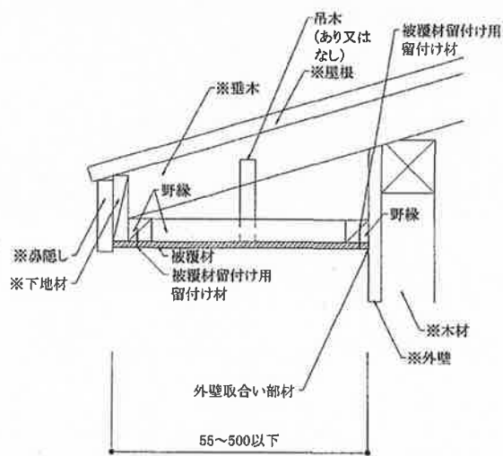
(水平軒/壁勝ち納まり)
