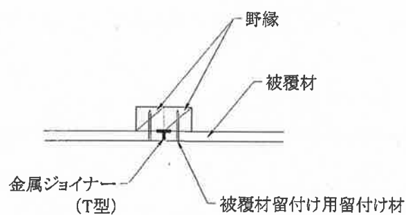
図4 構造説明図
