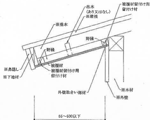
(勾配軒/被覆材勝ち納まり)
