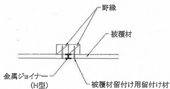
図4 構造説明図
