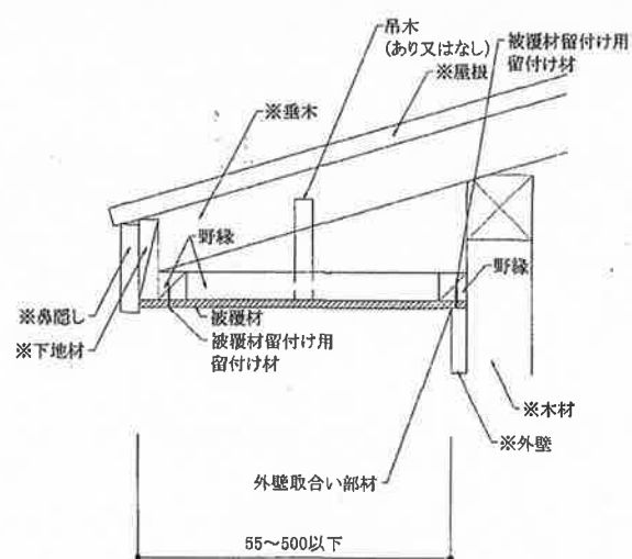
(水平軒/被覆材勝ち納まり)
