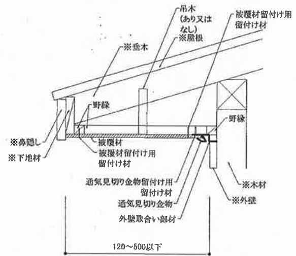
(水平軒/被覆材勝ち納まり)
