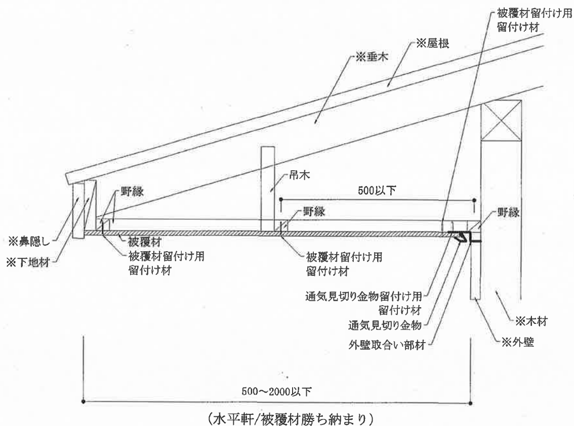
図 3 構造説明図
