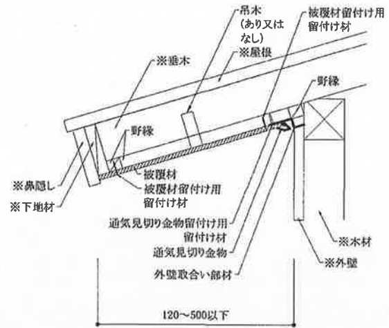
(勾配軒/被覆材勝ち納まり)
