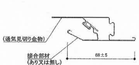
A図 接合部材形状図
