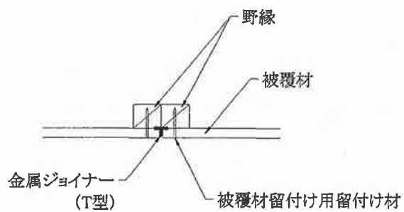
図4 構造説明図
