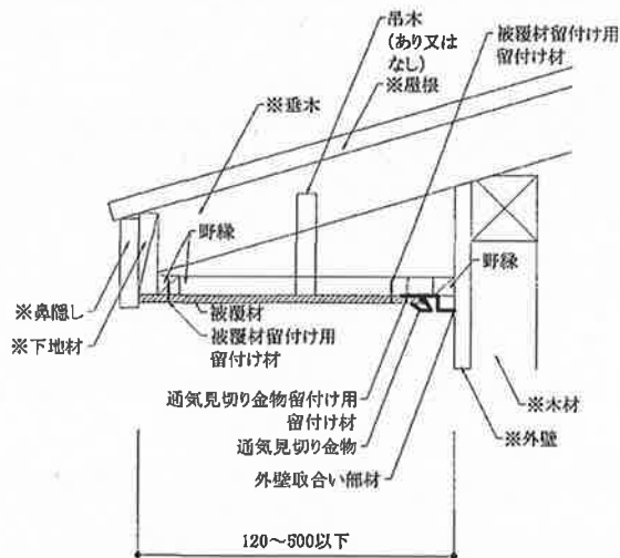
(水平軒/壁勝ち納まり)
