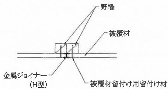
図4 構造説明図
