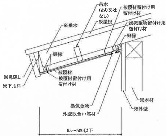
(勾配軒/壁勝ち納まり)
