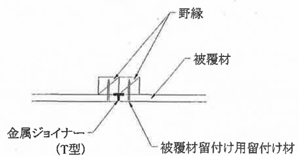
図4 構造説明図
