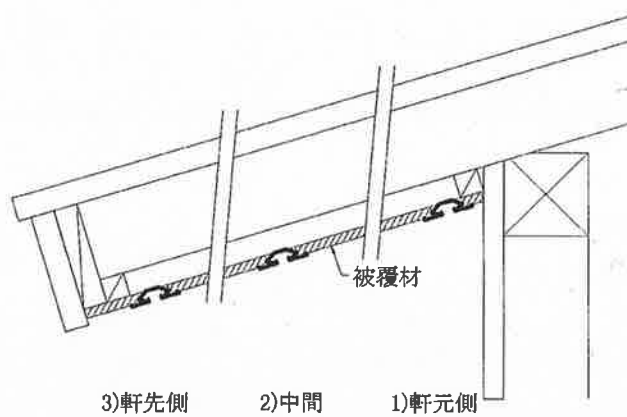
図5 構造説明図
