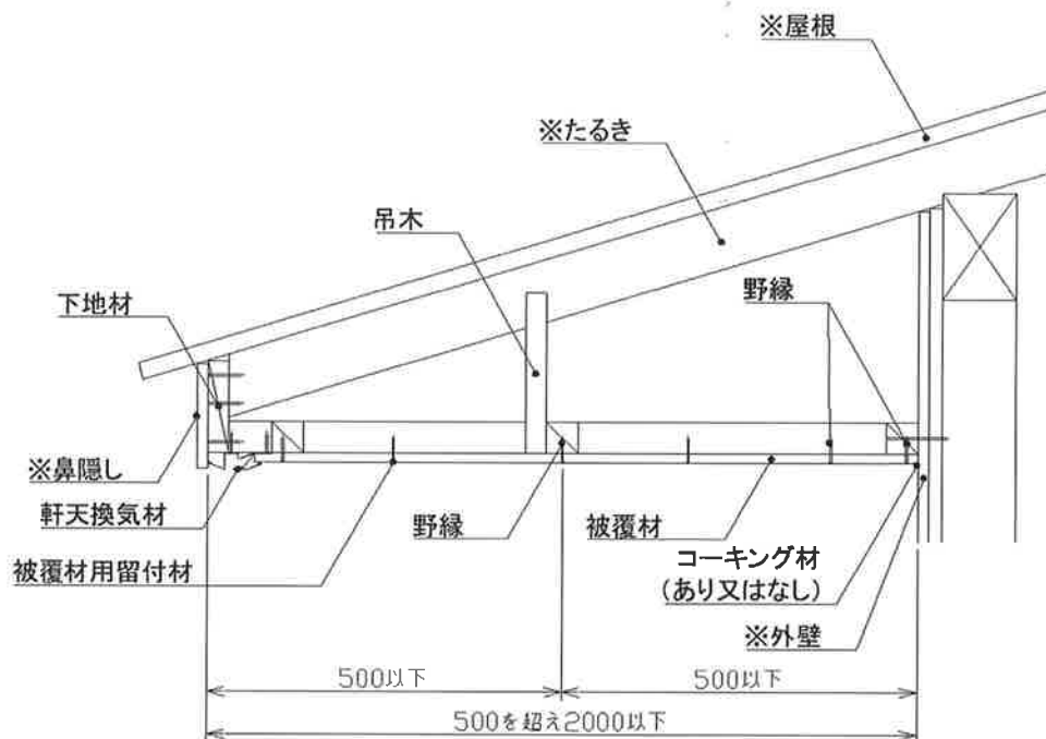
図 4 構造説明図
