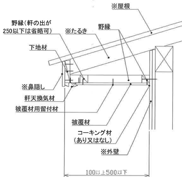
図 3 構造説明図
