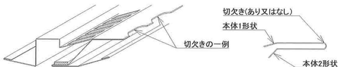
e) 鋼板非分割
