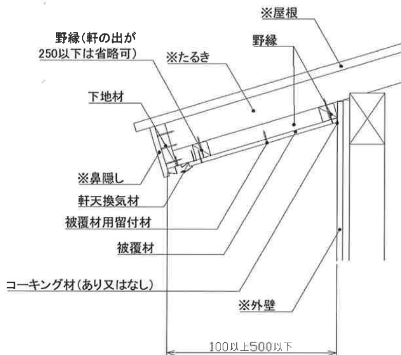
図 1 構造説明図
