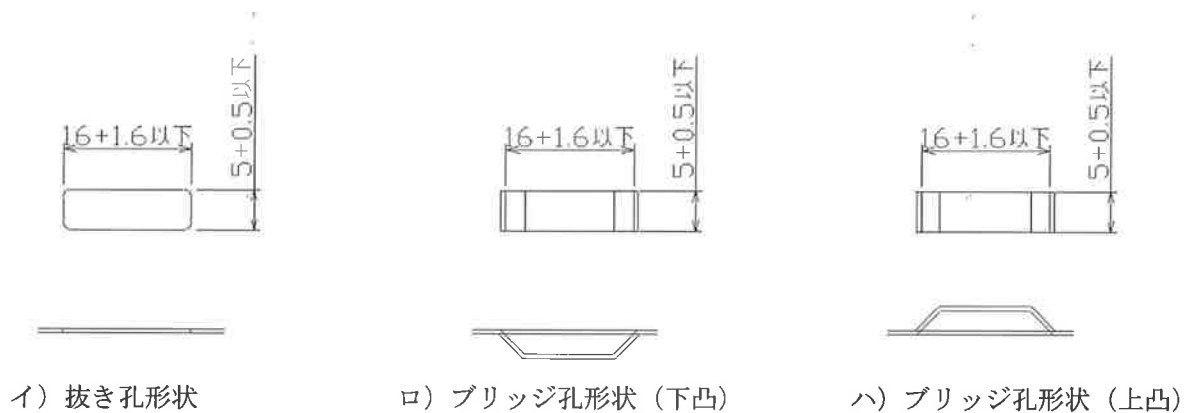
換気孔の形状図〔イ)～ハ)〕
