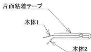
a) 本体固定部材片面テープ
