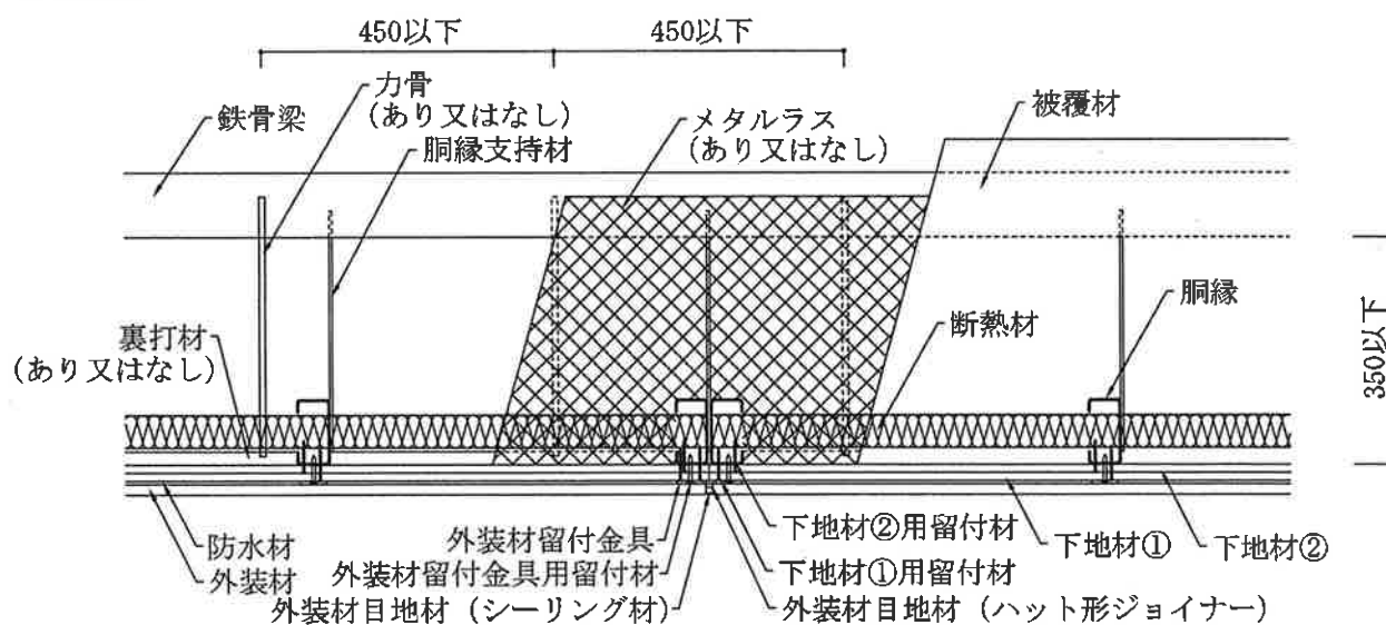
見上げ図
