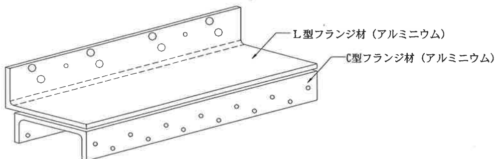
《制震ダンパー透し図》
