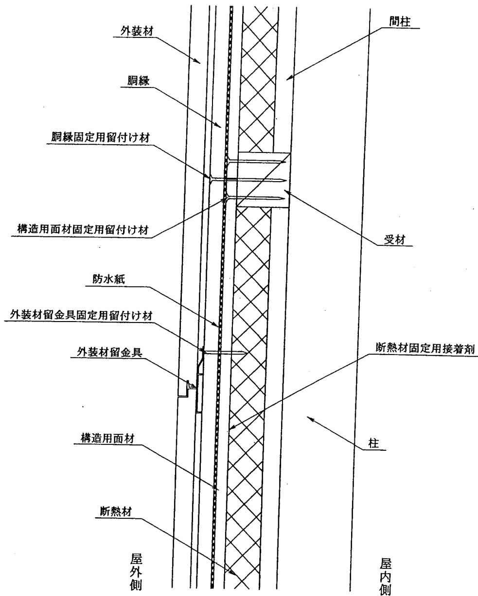
鉛直断面詳細図
