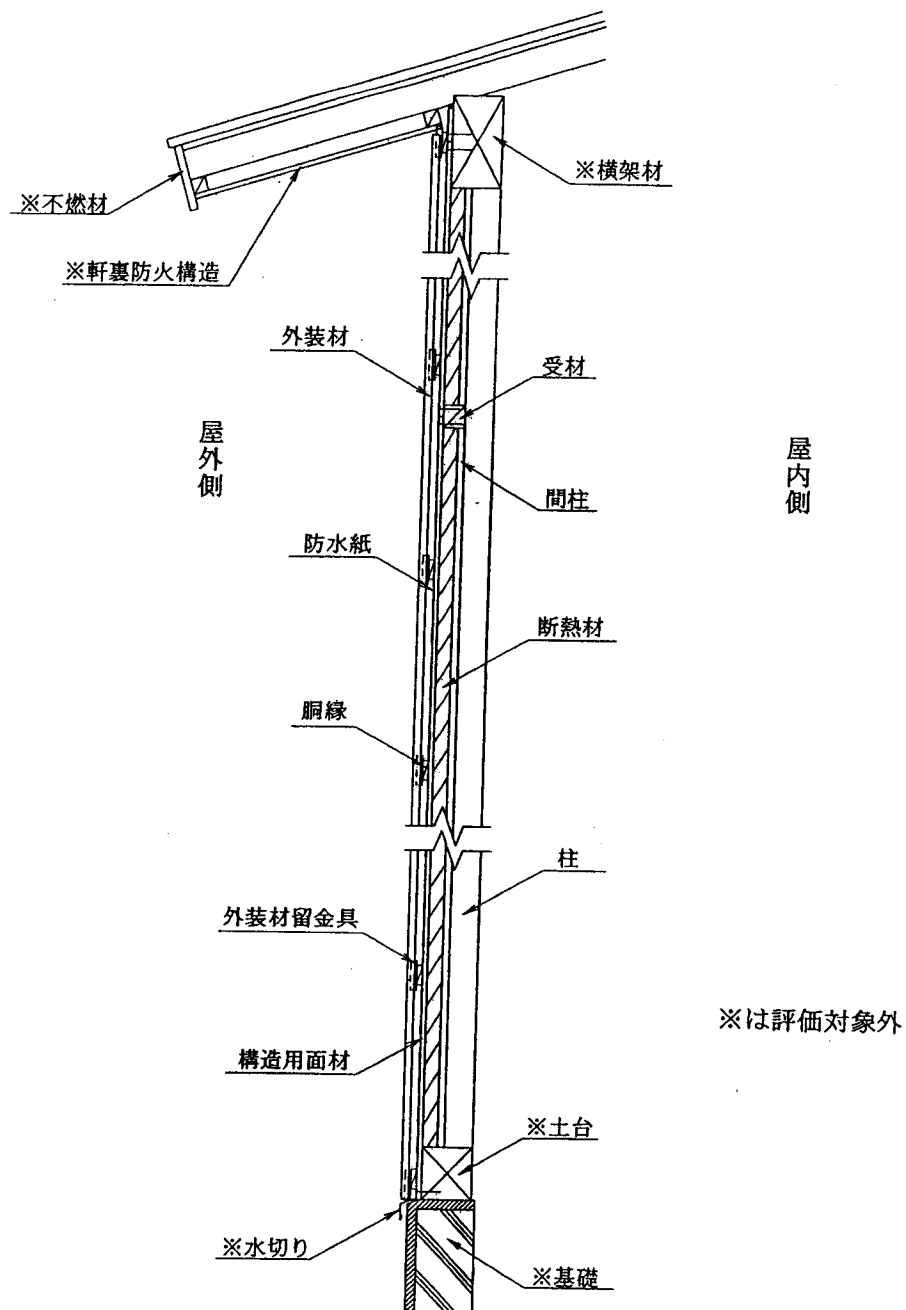
鉛直断面図
