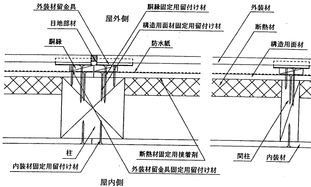
水平断面詳細図
