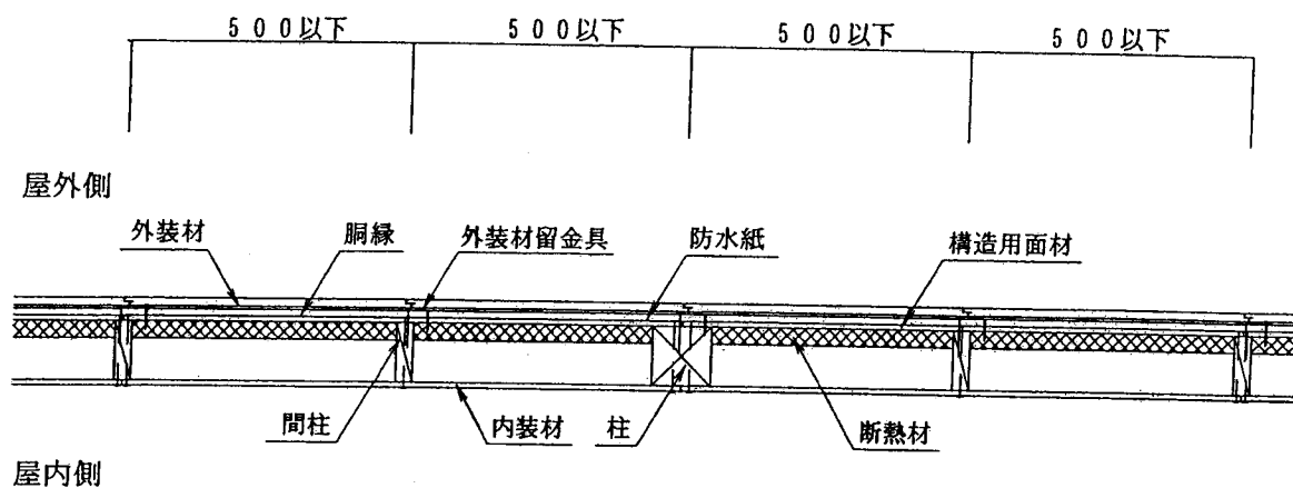
水平断面図
