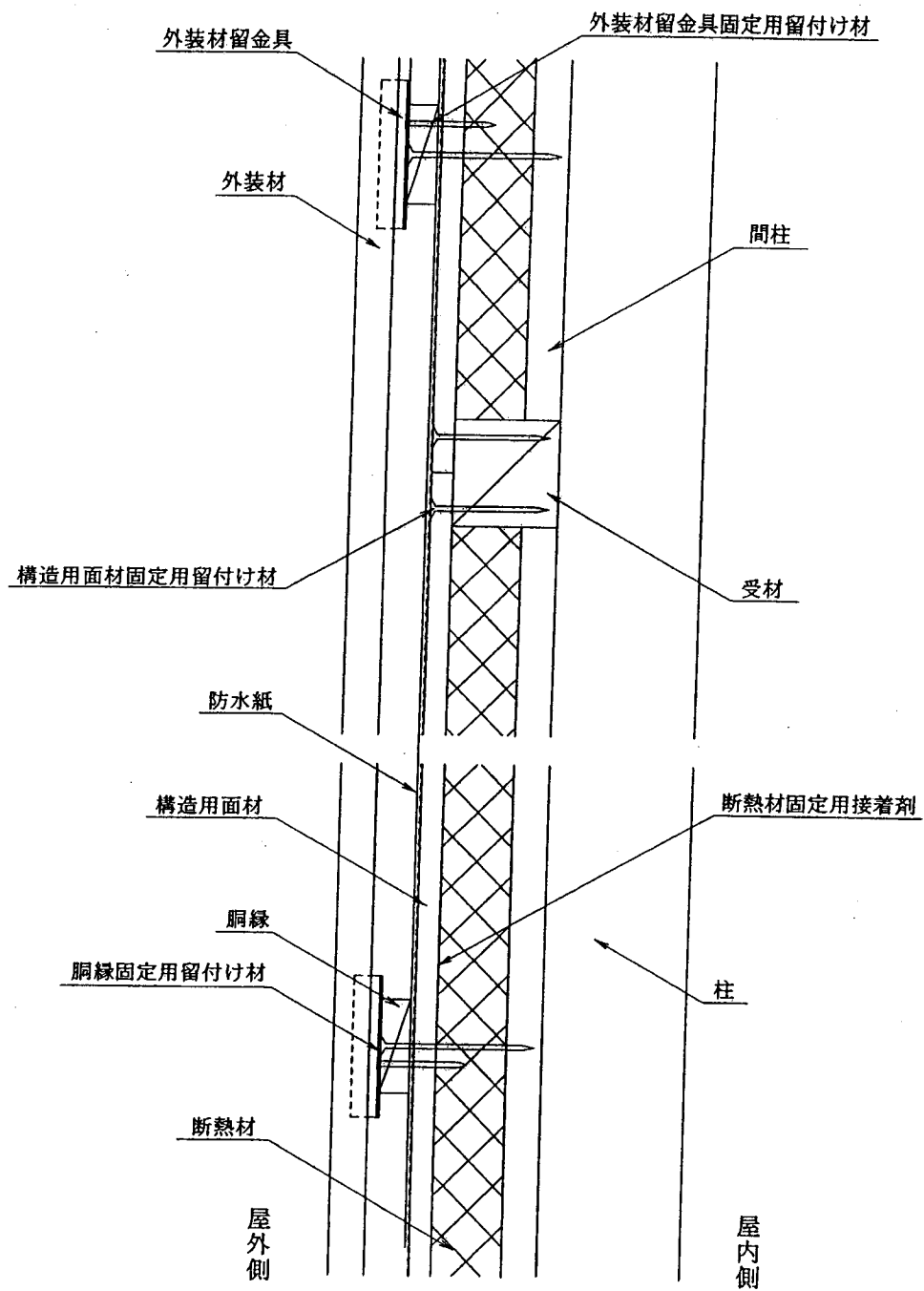
鉛直断面詳細図
