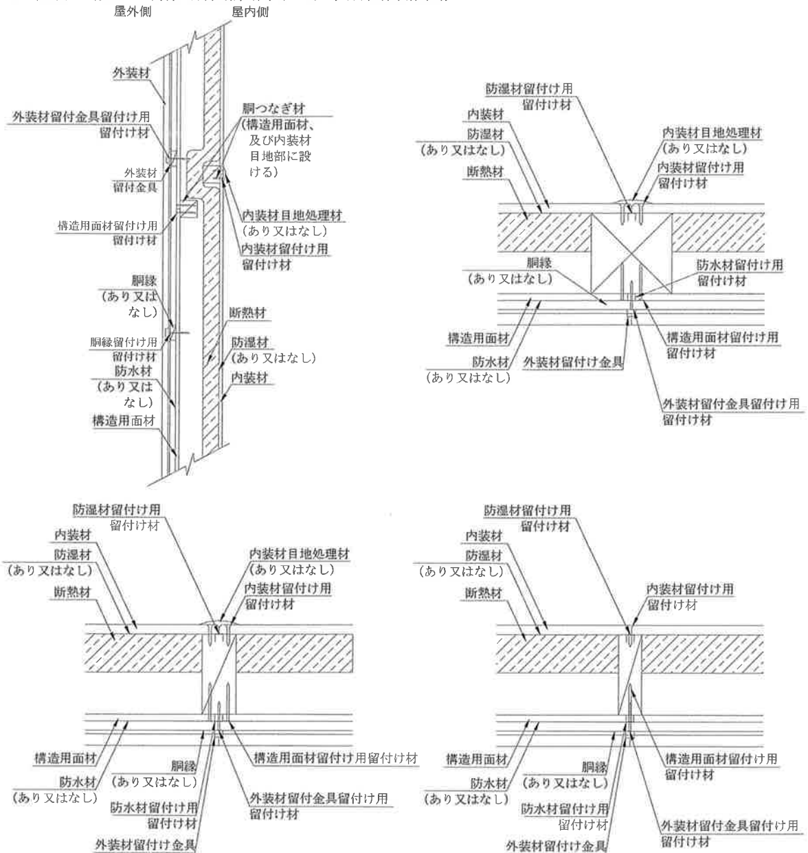
(外装材：縦張 鉛直断面詳細図 水平断面詳細図)
