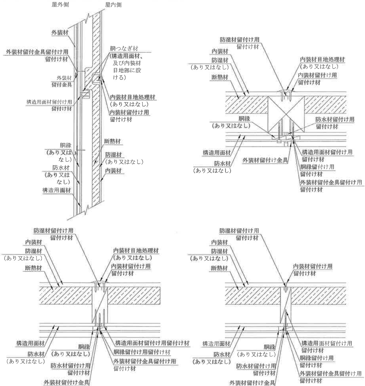
(外装材：横張 鉛直断面詳細図 水平断面詳細図)
