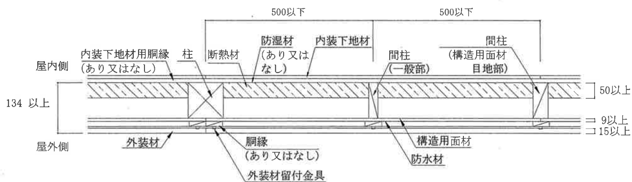
水平断面図
