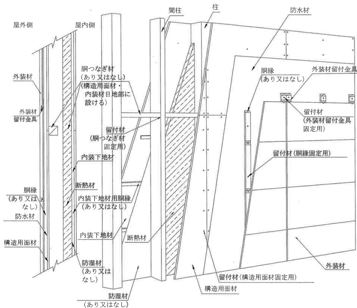
鉛直断面図
