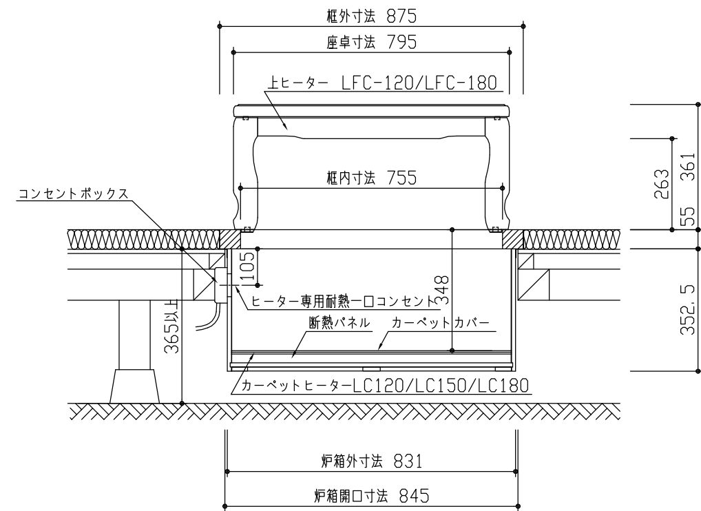
< オールシーズン炉箱 3×3尺タイプ >
