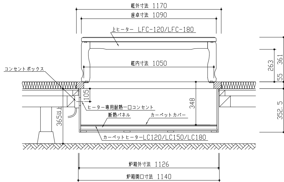
< オールシーズン炉箱 3×4尺タイプ >
