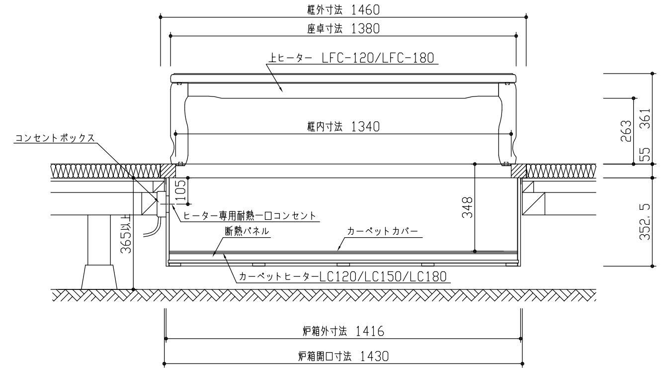
< オールシーズン炉箱 3×5尺タイプ >
