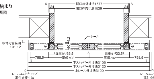
標準納まり
