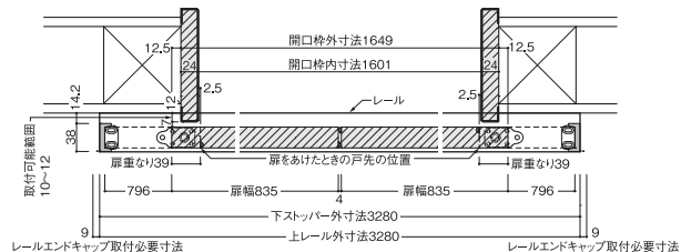
無目枠標準納まり 横断面図
