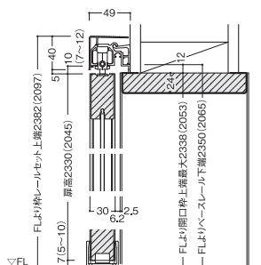
縦断面図 ※図は8尺高、( )は7尺高の場合
