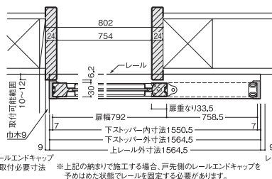
横断面図
