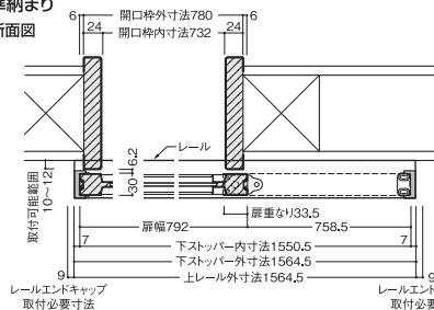
標準納まり
