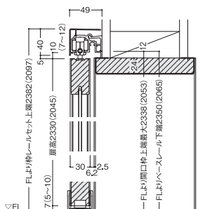
入隅納まり
