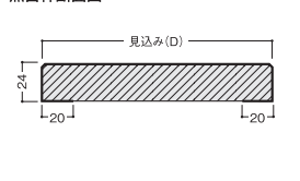
無目枠断面図
