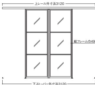
標準納まり
