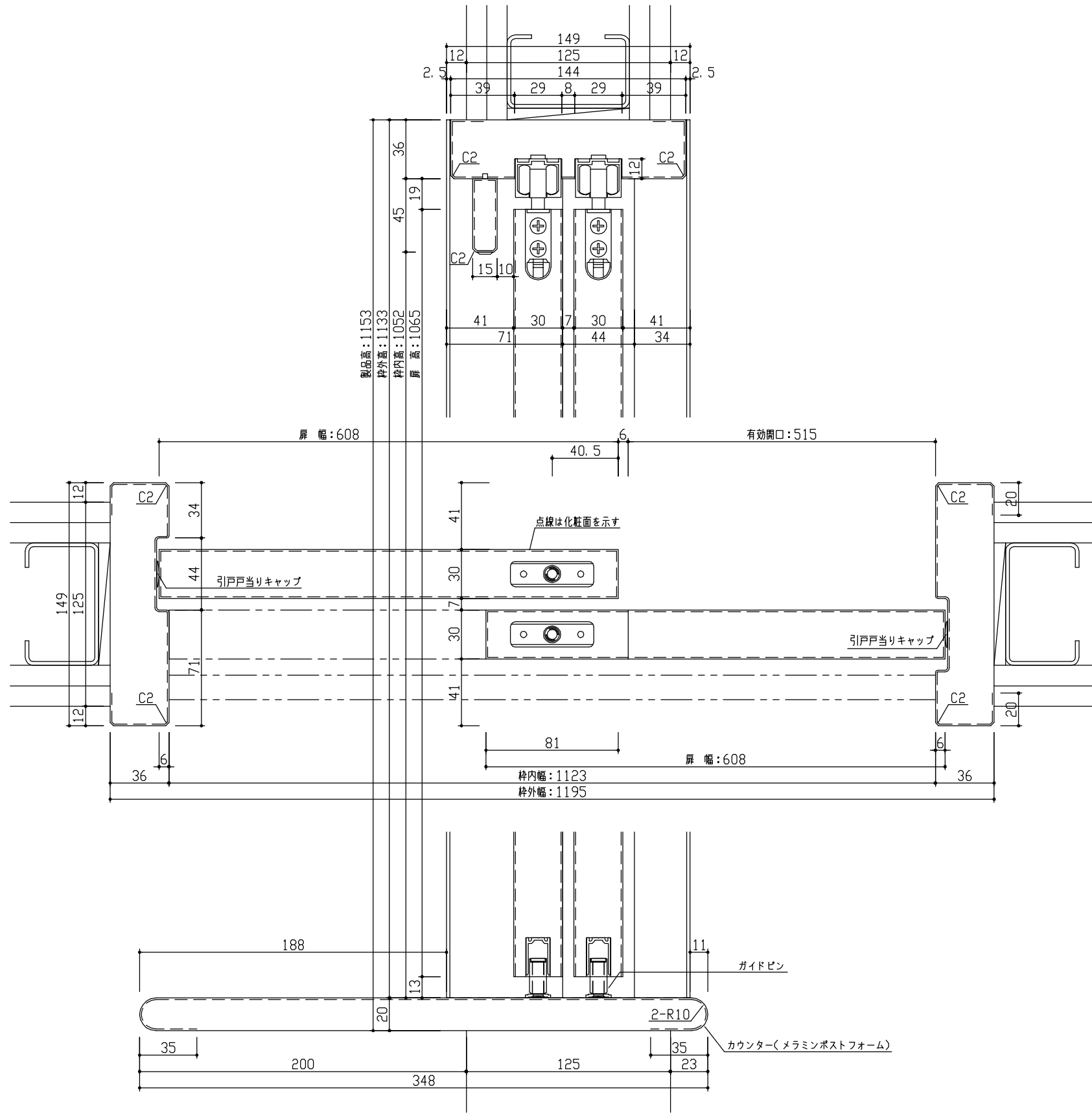
断面図
