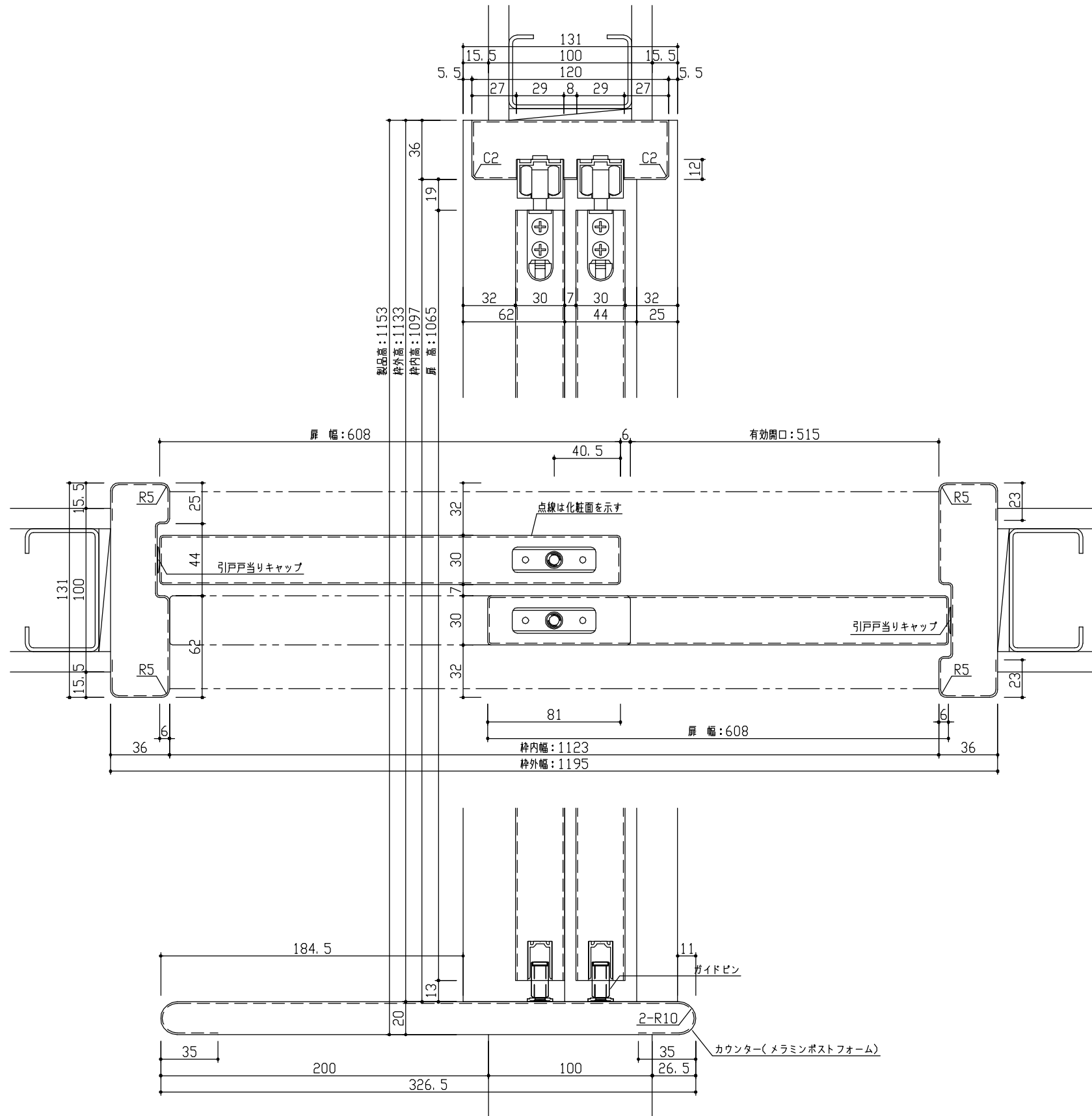
断面図
