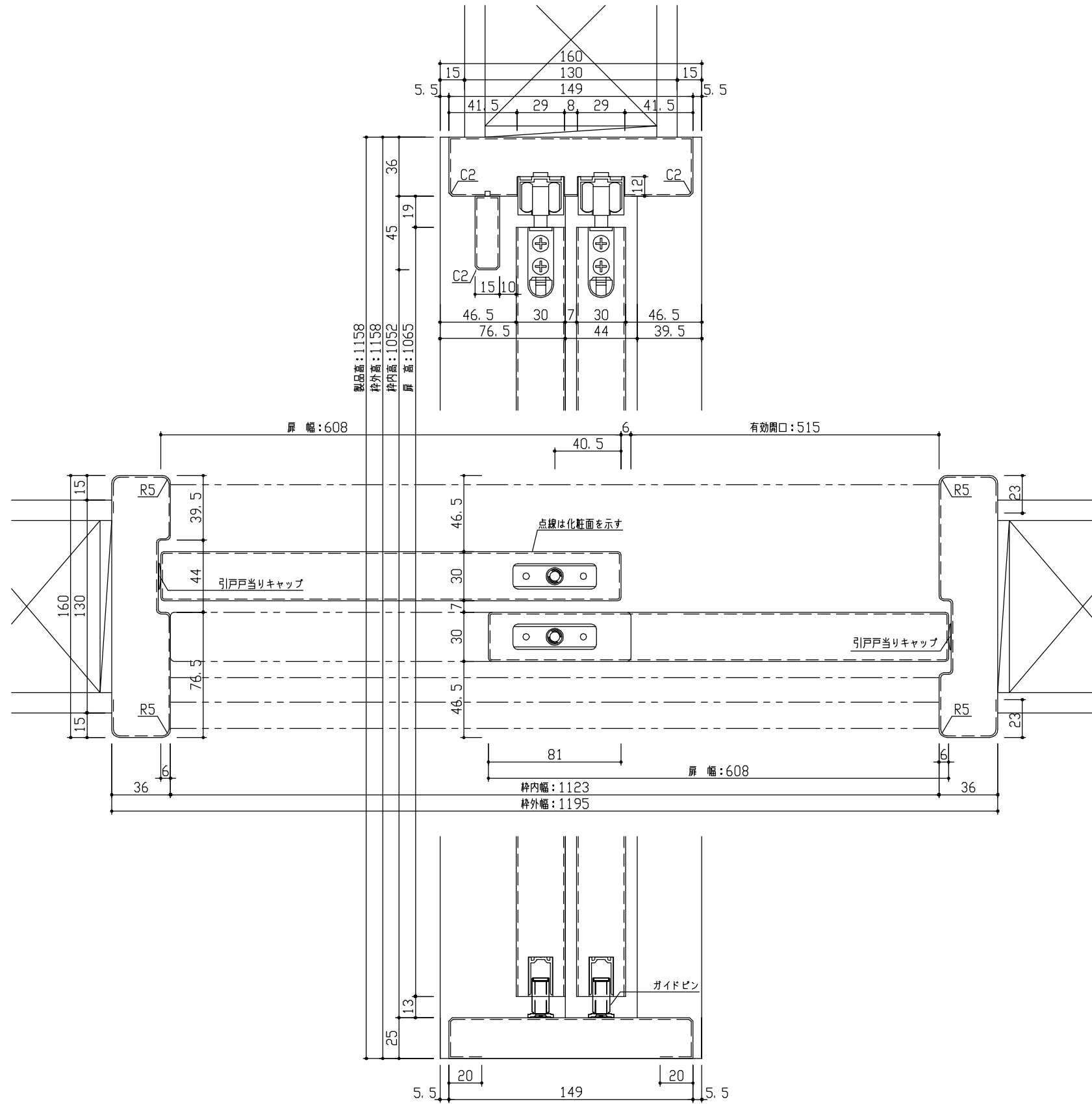
断面図
