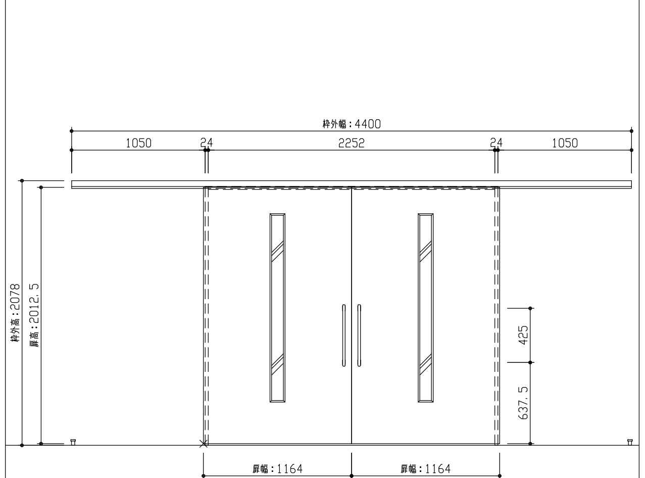
正面図
