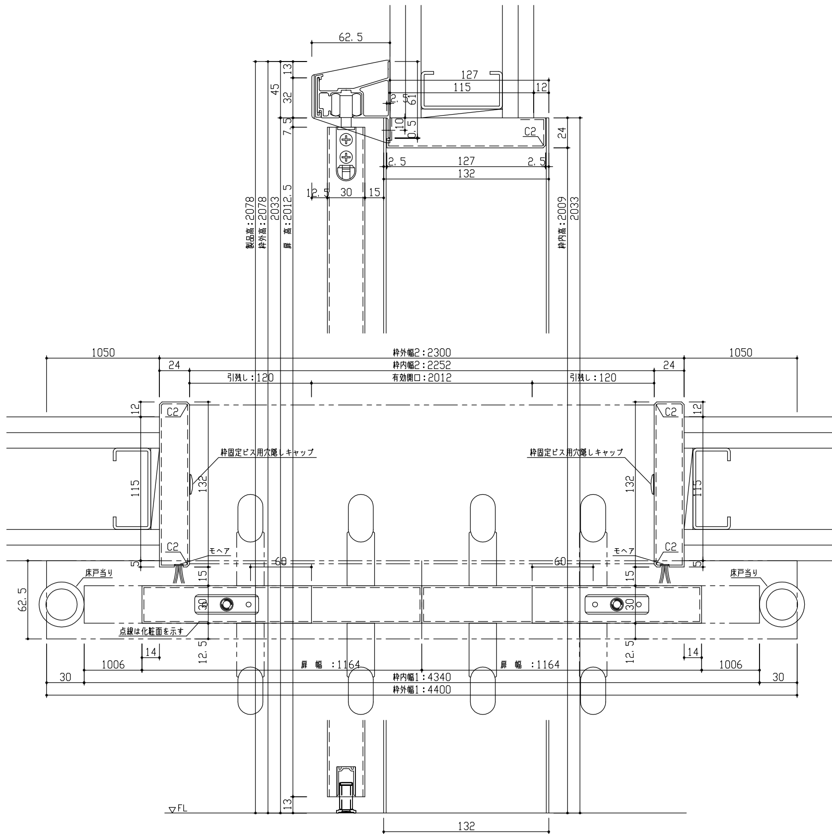
断面図
