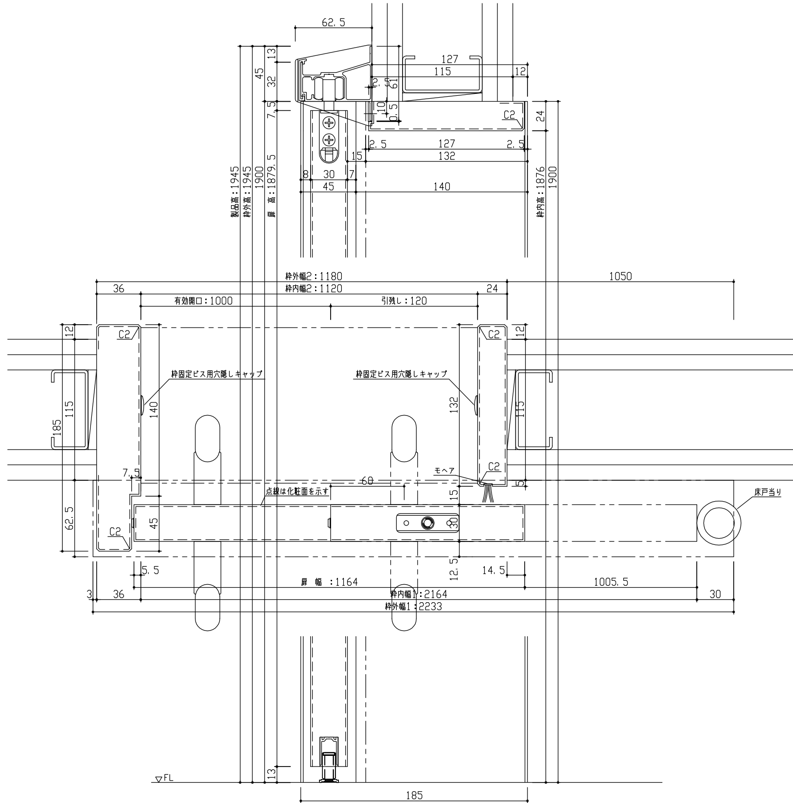
断面図
