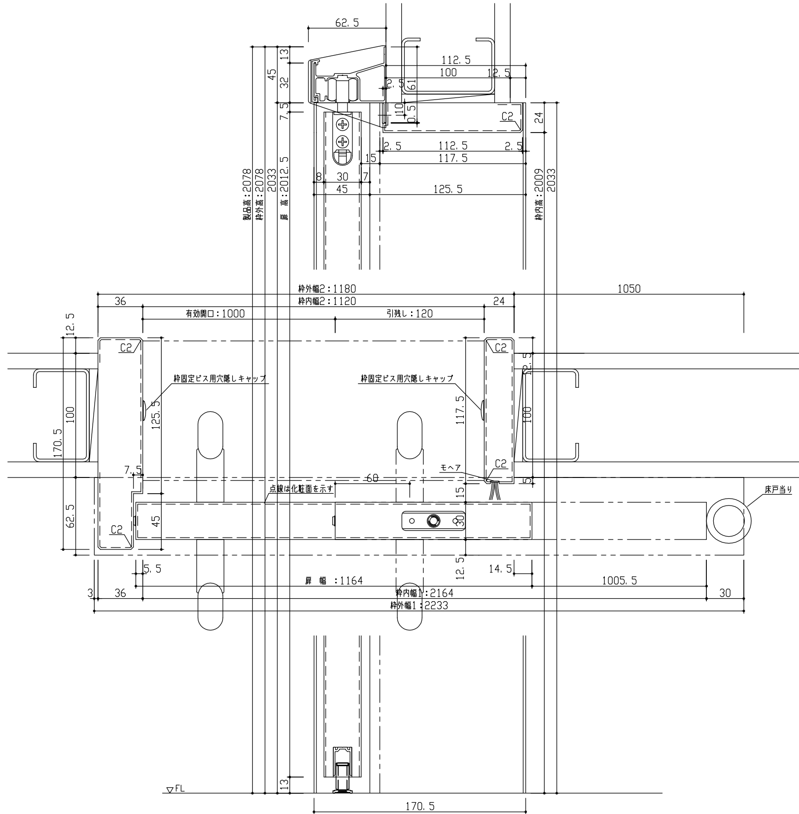
断面図
