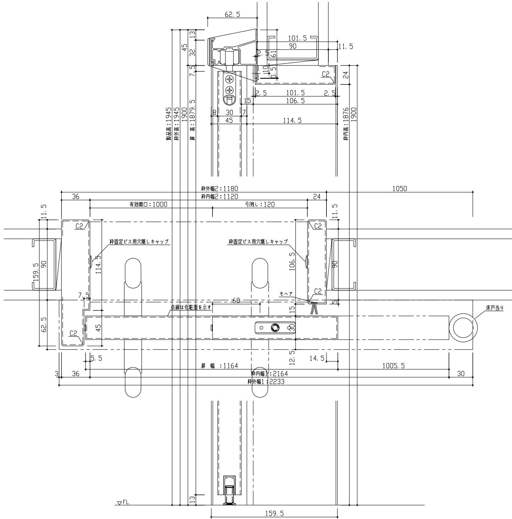
断面図
