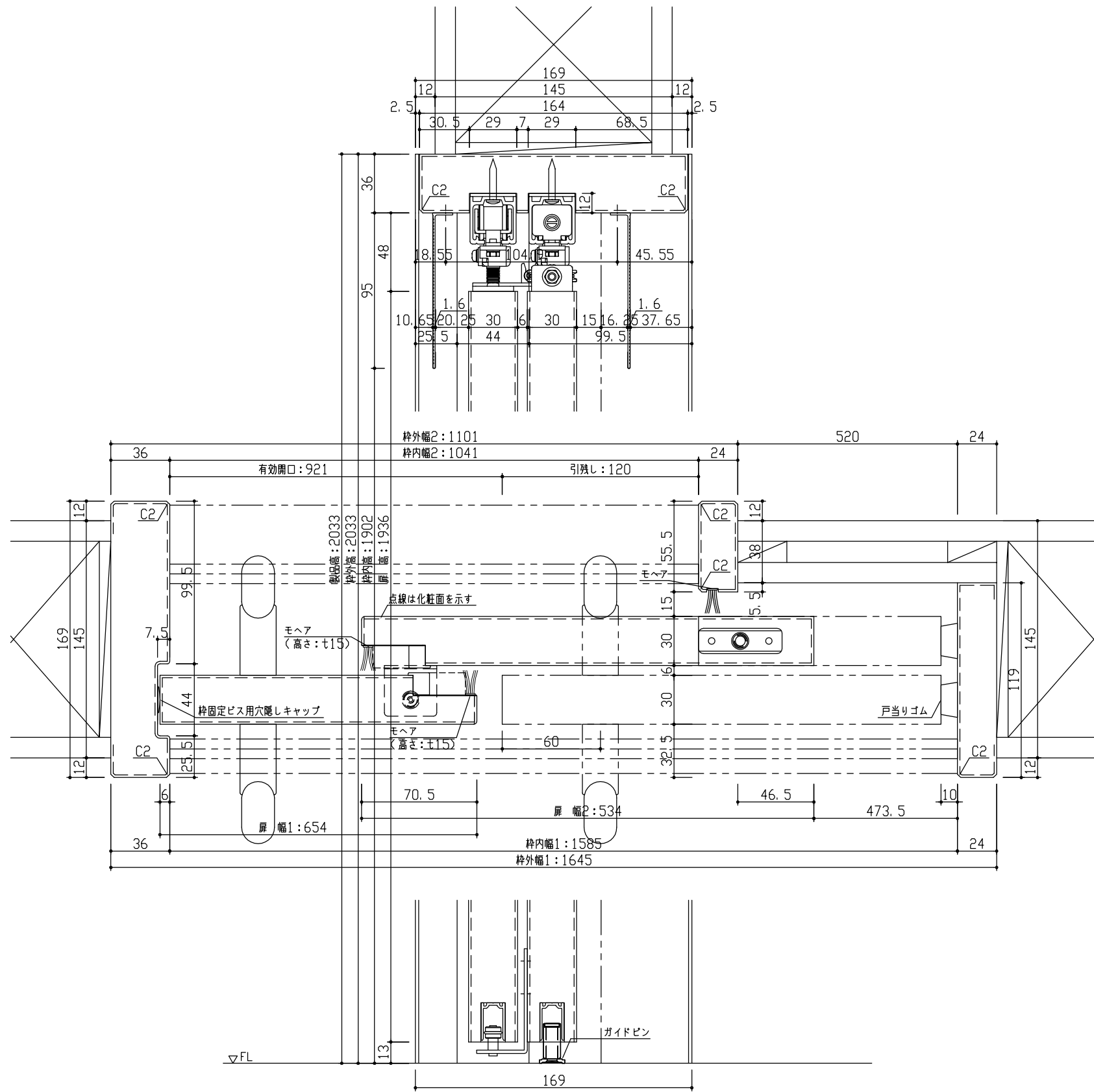
断面図
