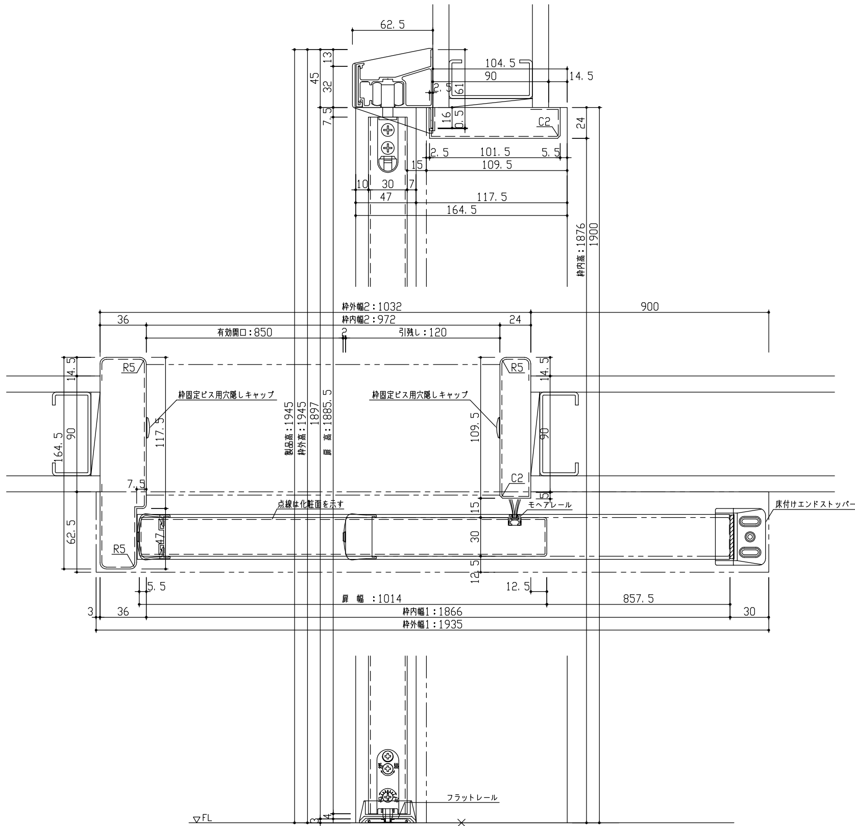
断面図
