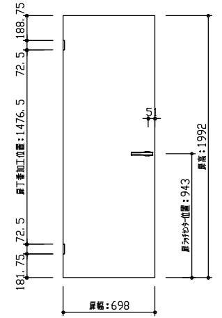
扉 正面図
