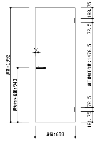
扉 正面図
