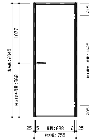
扉・枠 正面図
