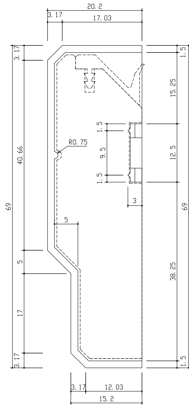
参考：ハンギング長押エンド部材納まり図
