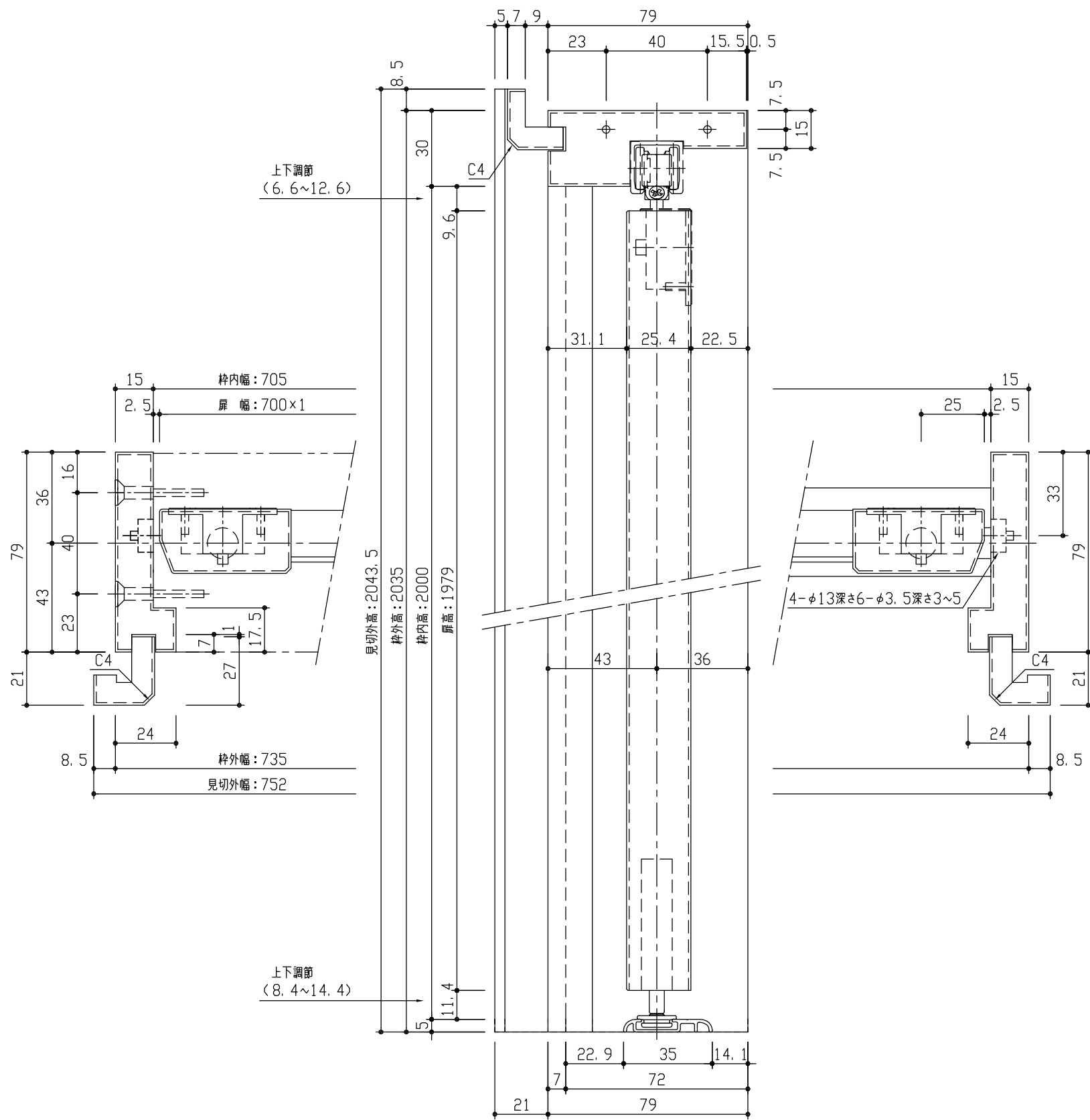
断面図
