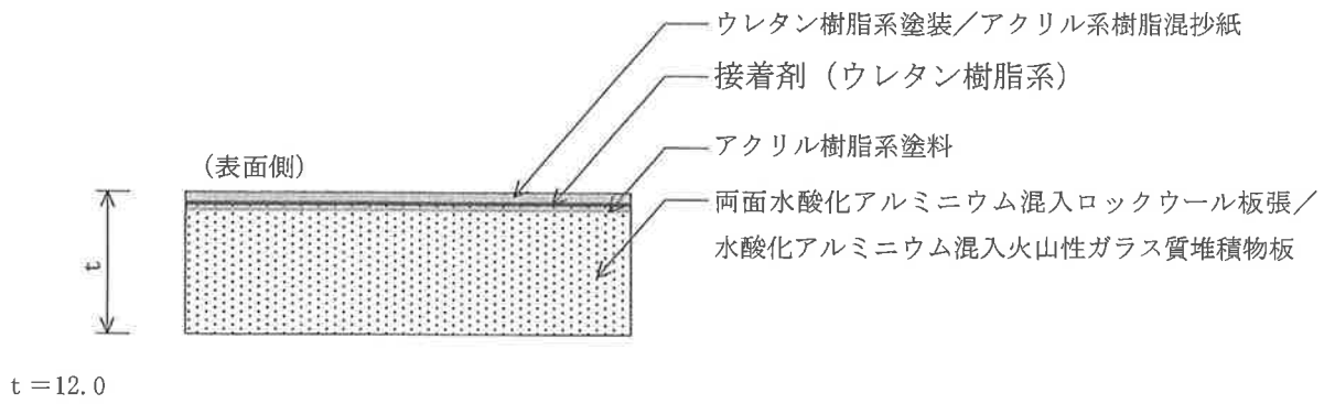
図1 断面図
