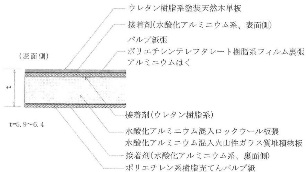
図1 断面図
