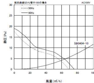
P-Q特性図
