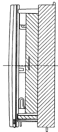
風向シャッター開時
