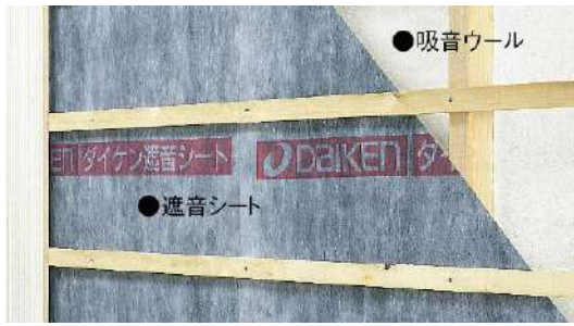
壁下地に『遮音シート』と『吸音ウール』を使用した施工例
