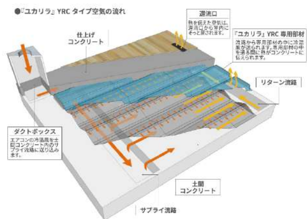
『ユカリラ YRC タイプ』システム概略図
