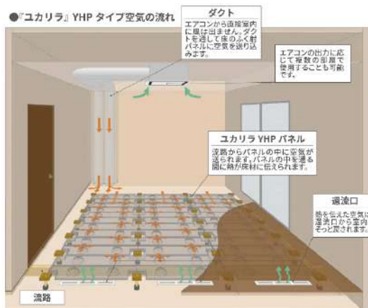
『ユカリラ YHP タイプ』システム概略図
