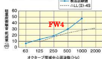
■床衝撃音レベル低減試験結果
