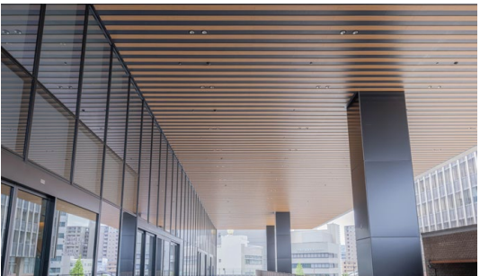
軒天井材 (屋外)：ダイライト 軒天羽目板 (特注品) 天井造作材 (屋内)：グラビオールバー UB 直付式 (特注品)
