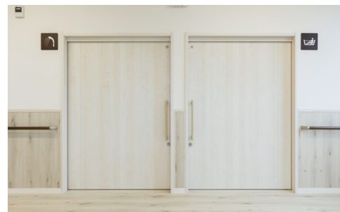
室内ドア：おもいやりドア〈ネオホワイト柄〉 手摺：システム手摺35型 ゴム集成材タイプ手摺〈ダルブラウン色〉
