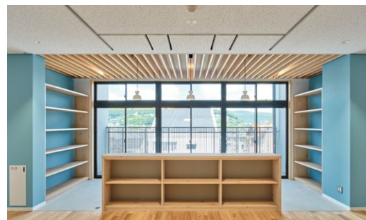
天井造作材：グラビオルーバー US 直付式〈三次市産杉〉 床材：コミュニケーションタフII DW〈アッシュ (クリア色)〉
