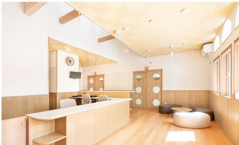
室内ドア：おもいやりキッズドア〈ライトオーカー柄〉 腰壁：ハピアウォール ハードタイプII〈ライトオーカー柄〉 床材：コミュニケーションタフII DW〈ハードメープル〉 天井材：パステルトーン〈イエロー色〉
