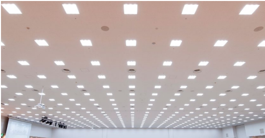
耐震天井工法：ダイケンハイブリッド天井 天井材：ロックウール化粧吸音板 ダイロートン トラバーチン12mm
