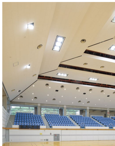
耐震天井工法：ダイケンハイブリッド天井 天井材：ロックウール化粧吸音板 ダイロートン ワイド直張〈トラバーチン〉
