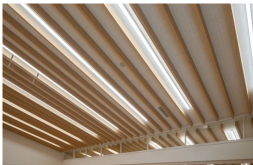
天井造作材：グラビオルーバー UB 直付式〈UB15〉 天井材：クリアトーン9ラインアート〈402〉
