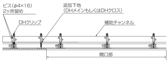
D-D断面
