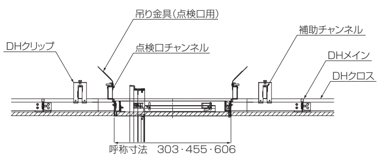
I-I 部分断面図
